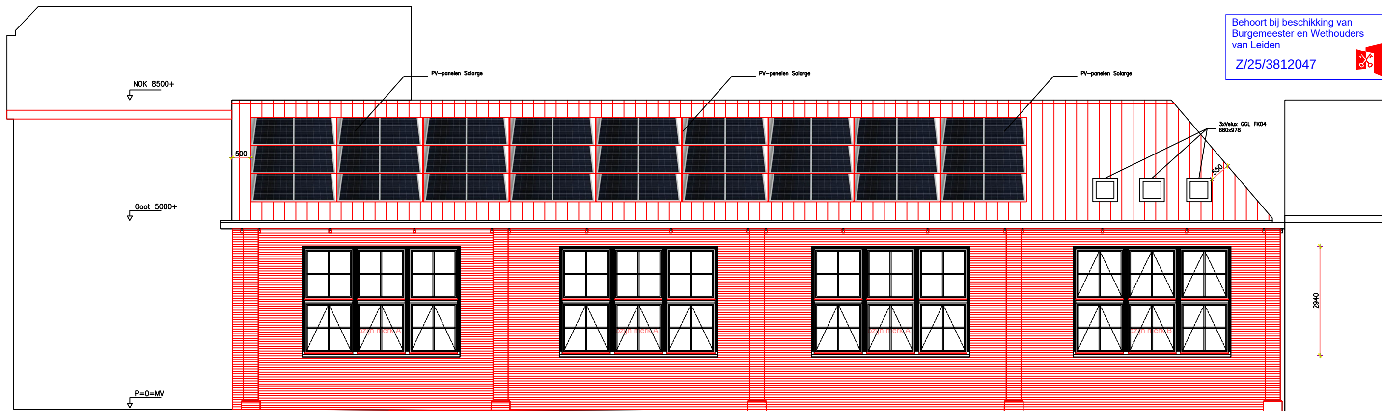
Gevelaanzicht Pioenstraat
